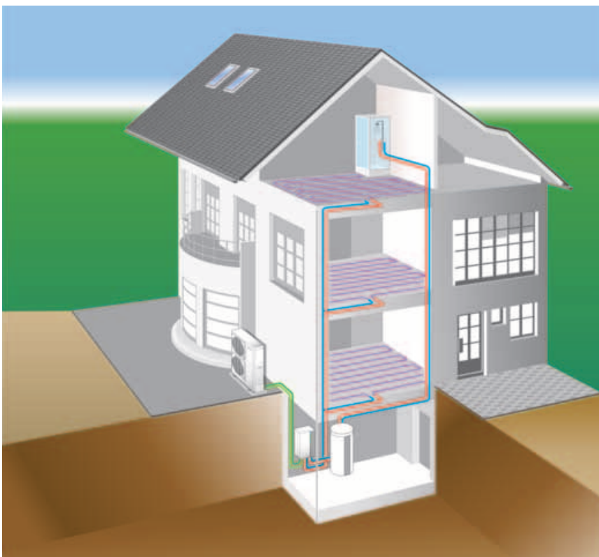
Luft/Wasser-Wärmepumpe Split
