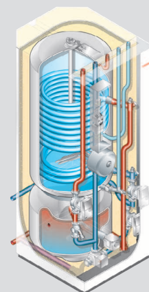
Kombispeicher WKS
