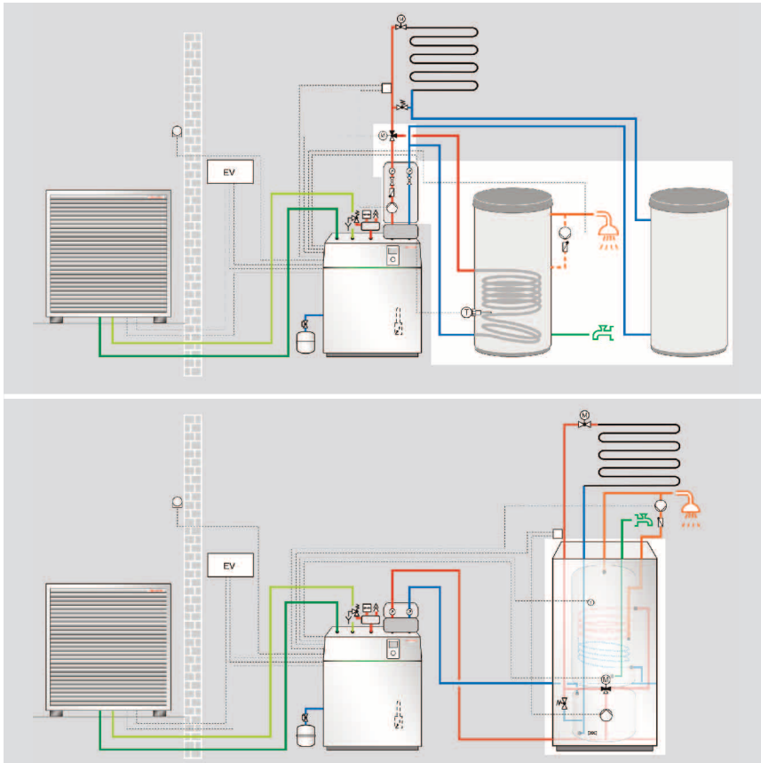
Vergleich einer Wärmepumpeninstallation ohne und mit Weishaupt Kombispeicher WKS / C
