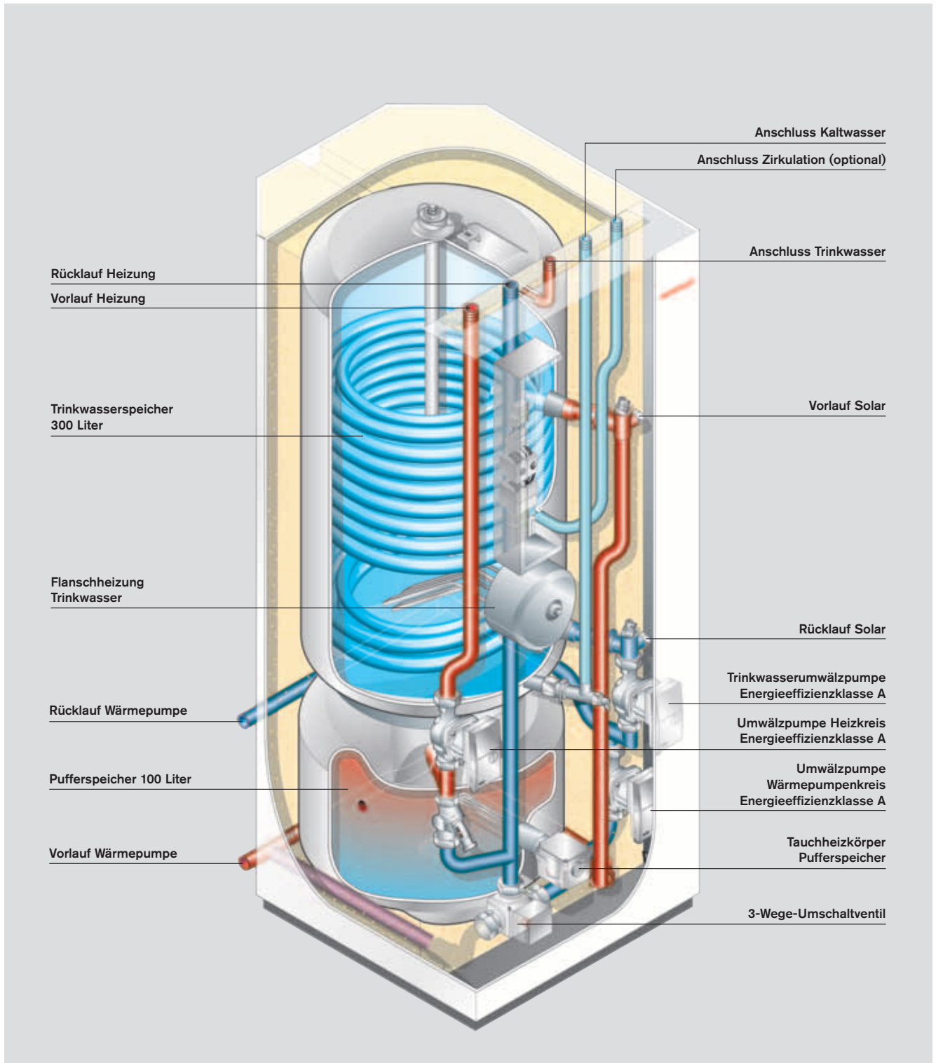
Weishaupt Kombispeicher WKS 300 / 100 LE / Unit-E / Bloc / B für Monoblock-Wärmepumpen
