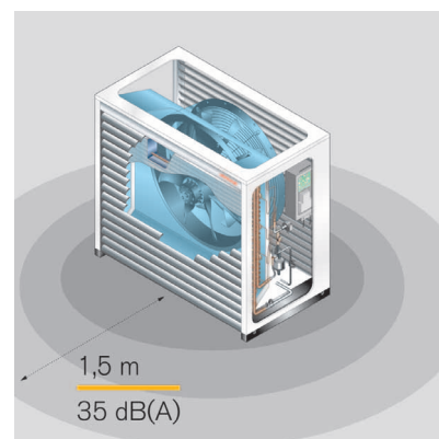
Beispieldarstellung: das Aussengerät der WBB 12
